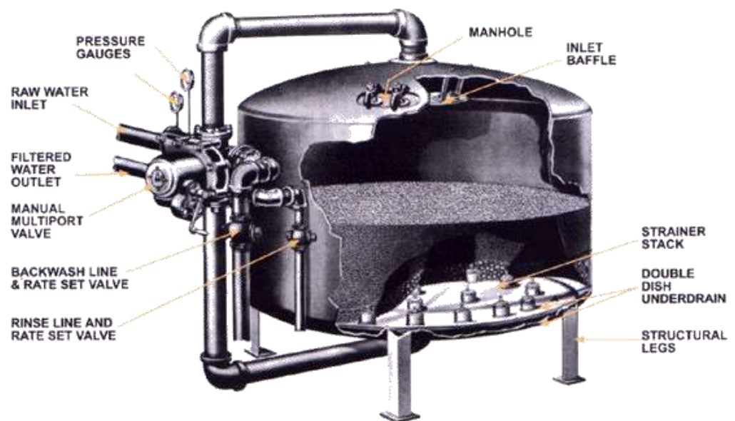
شکل فیلتر سنی فشاری
